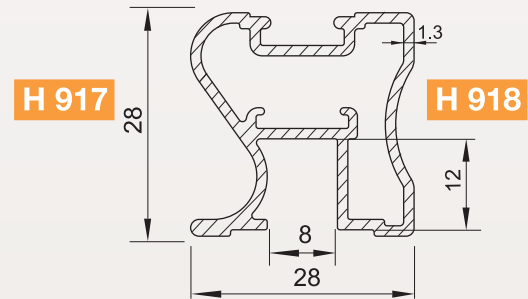
H 917 / H 918 Yan (kulp) Profil Side (handle) Profile
