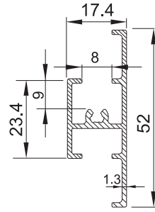
H900-GA Geniş Ara Profil / Wide Range Profile H911 Ürünlerinde Kullanılır / Used in Products
