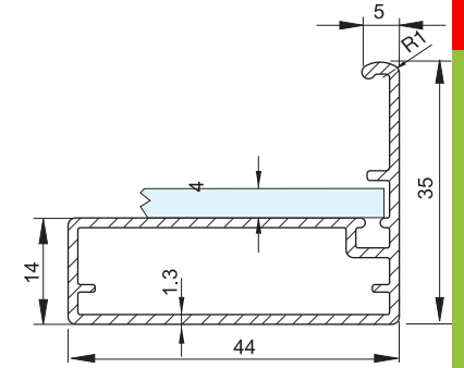
H880 Boy Kulp Kenar Kapama Length Handle Edge
