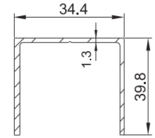
H900-TÜR Tekli Üst Ray / Single Upper Rail
