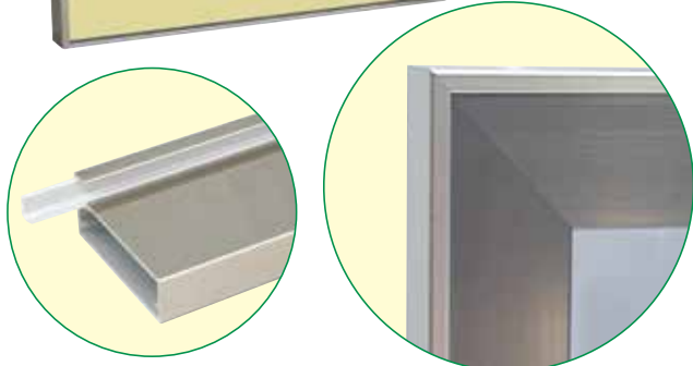
Köşe birleşme detayı Corner joint detail
