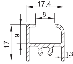
H900-ÜR Üst Ray / Upper Rail
